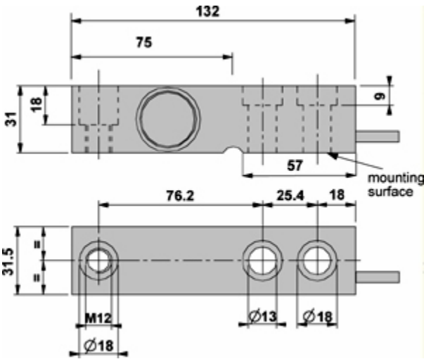
Dimensiones (mm)
